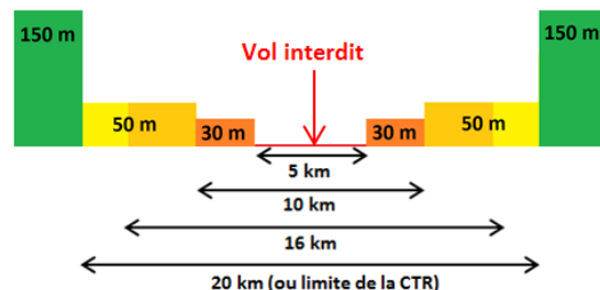
Vues transversales
